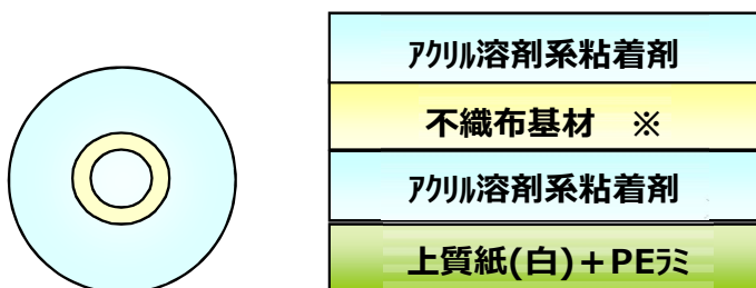
図. ND-2330SP テープ構成
